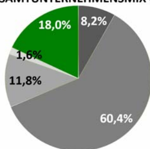
GESAMTUNTERNEHMENSMIX GWP
